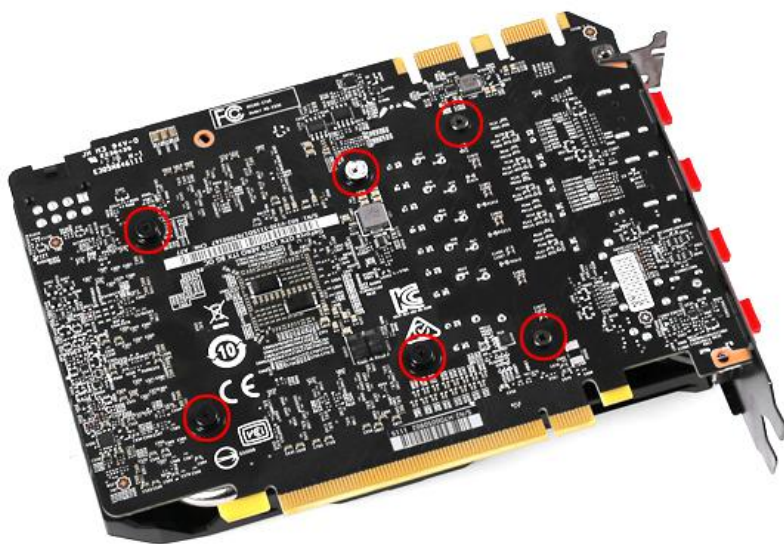
1. 拆除图中标红位置螺丝
