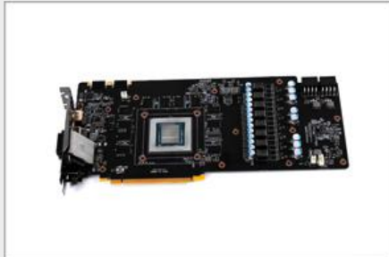
清理并重新涂抹导热硅脂
