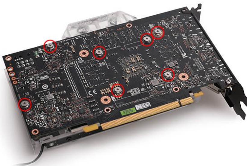
6.安装图中标红位置螺丝
