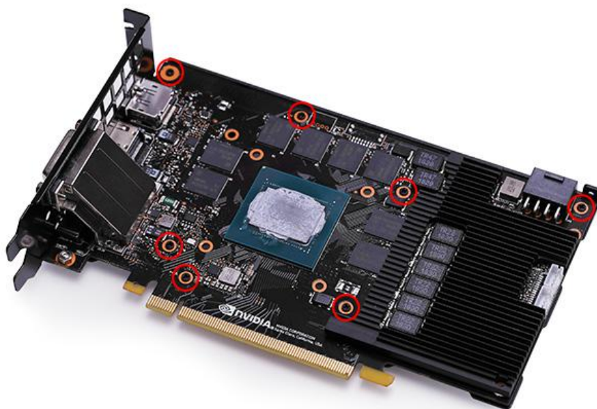
2. 拆除图中标红位置螺丝
