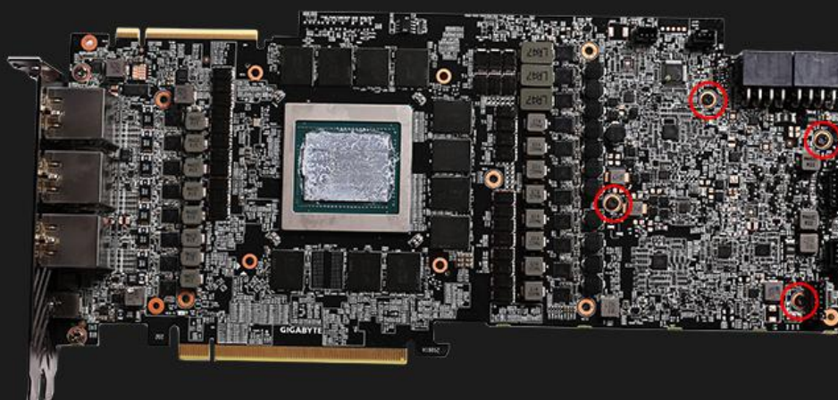
2. 拆除图中标红位置螺丝
