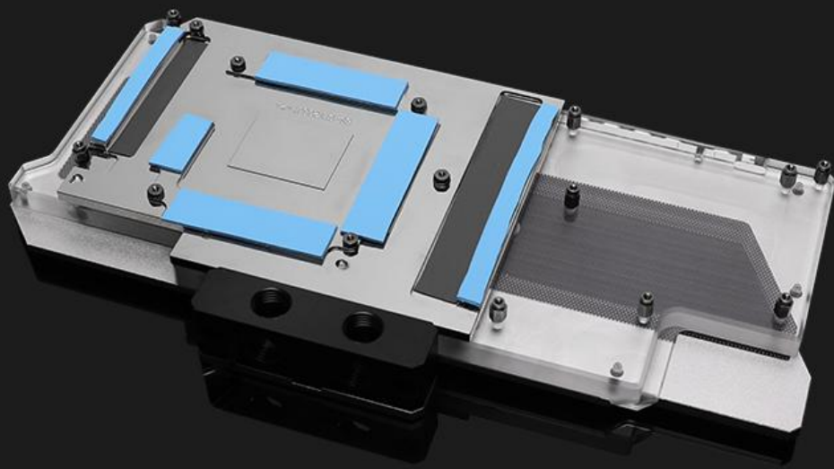
4.在相应位置贴好相应规格导热硅脂条，注意剪切尺寸
