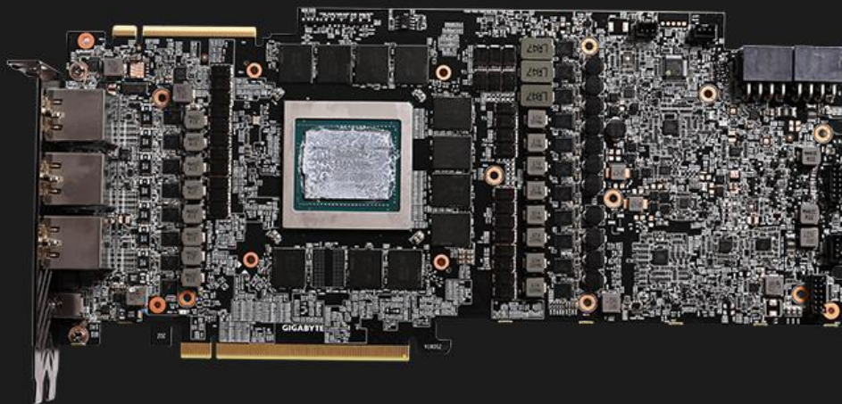
3.清理并重新涂抹导热硅脂
