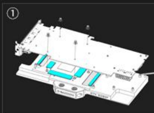
将显卡冷头底板螺丝对准显卡螺丝孔位使两者贴合
