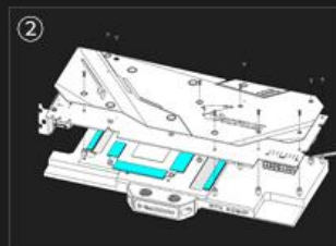
显卡原装背板孔位对准贴合用弹簧螺丝锁紧
