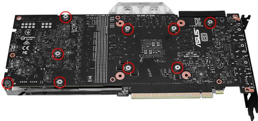
5.安装图中标红位置螺丝
