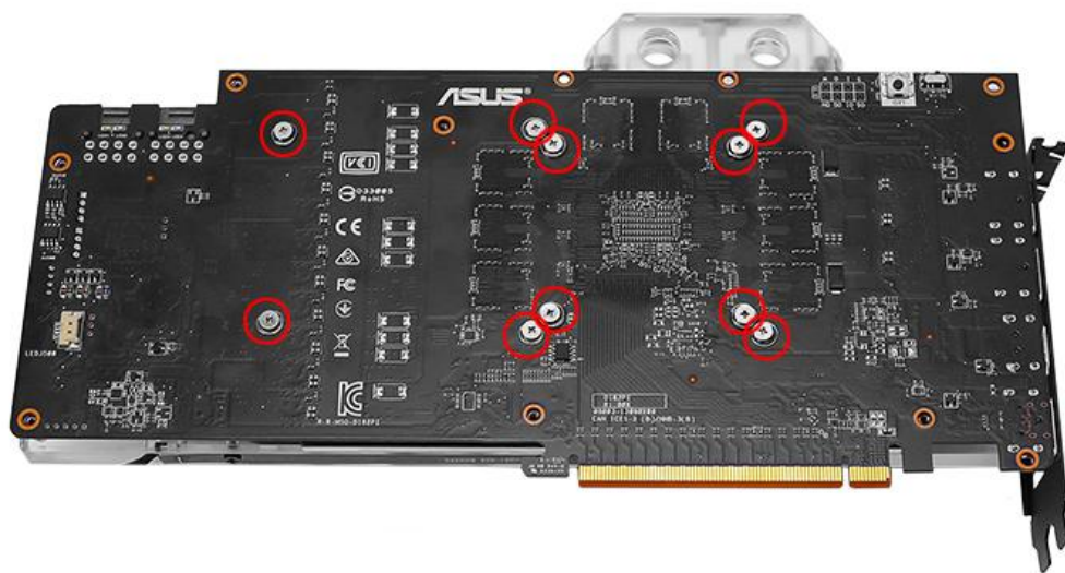
6.安装图中标红位置螺丝
