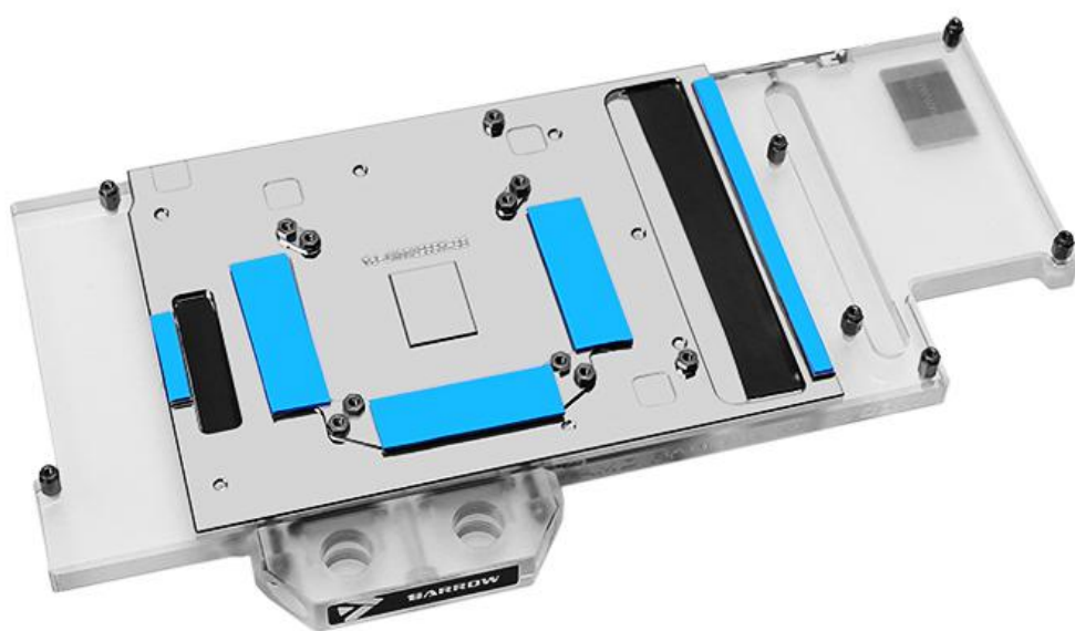
5.在相应位置贴好相应规格导热硅脂条，注意剪切尺寸
