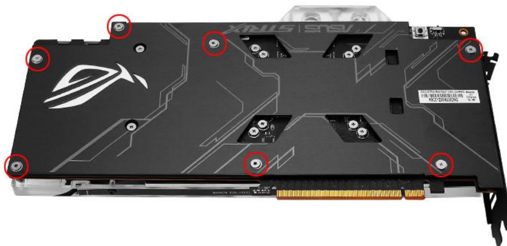
7.安装图中标红位置螺丝
