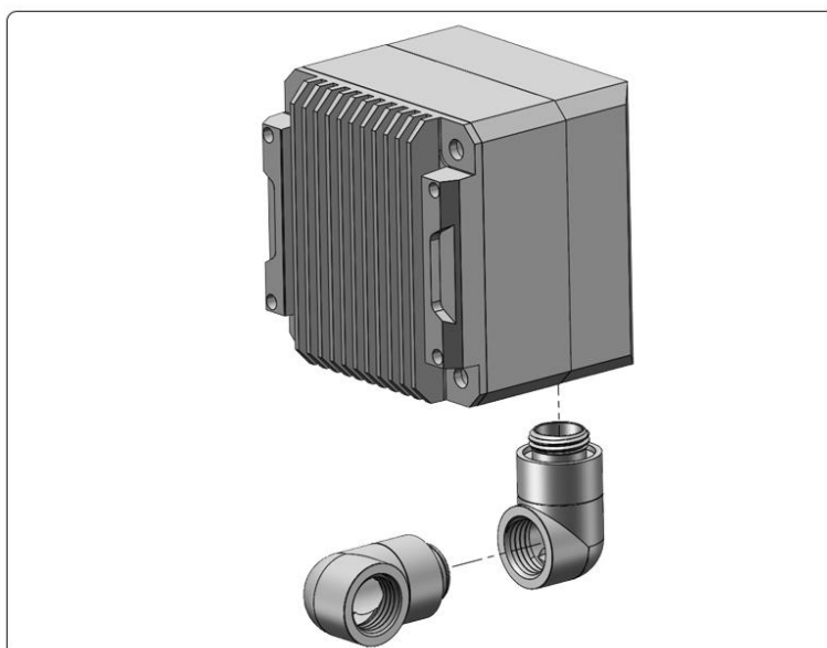
12.水泵装好接头
