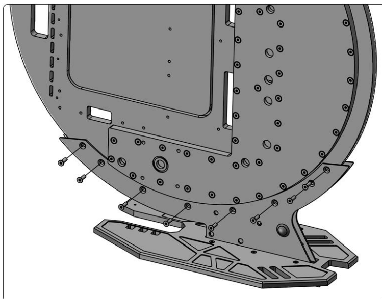
3.固定机箱主体
