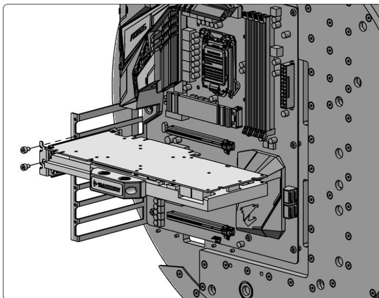
8-3.固定显卡
