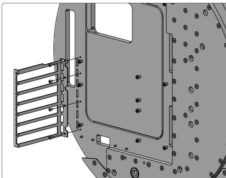
8-1.固定显卡支架
