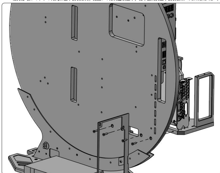
7-2.固定显卡竖装模块
