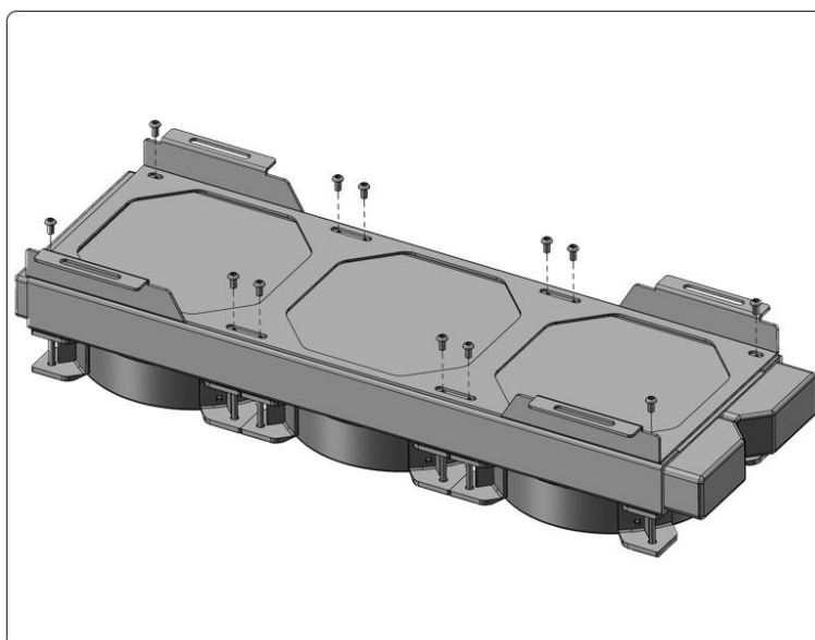
10.冷排与冷排支架固定
