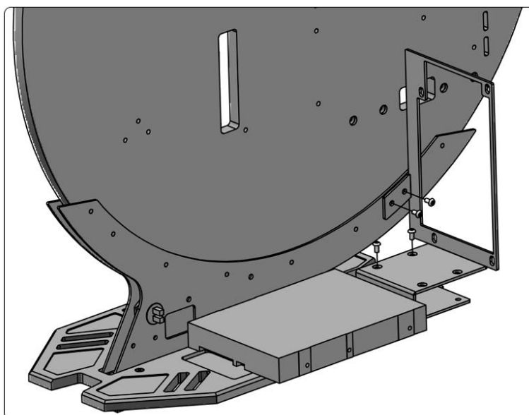
5.固定电源支架
