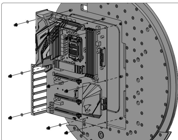
8-2.固定主板
