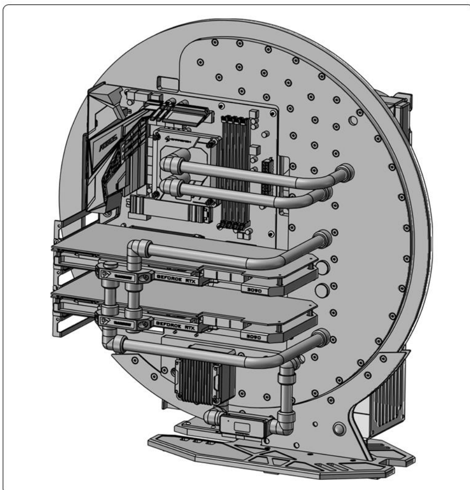
15. 安装完成
