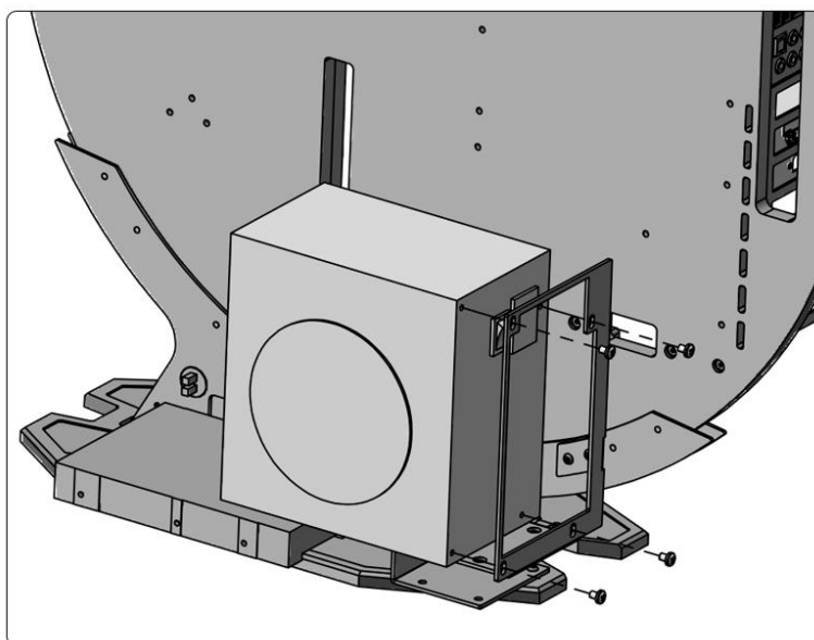
9.固定电源
