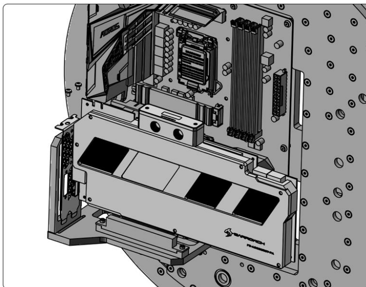
7-3.固定显卡
