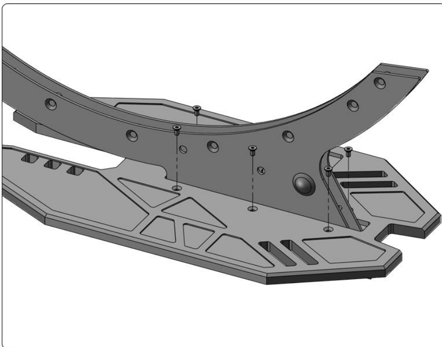
2.使用螺丝固定支架与底座
