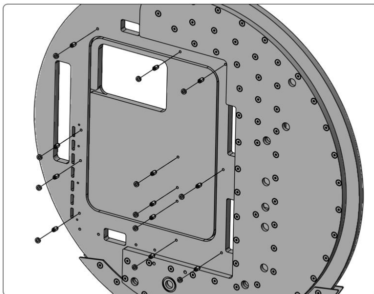
6.安装主板固定铜柱及ABS垫片
