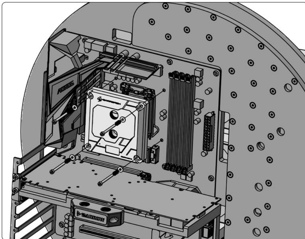
14. 安装CPU冷头
