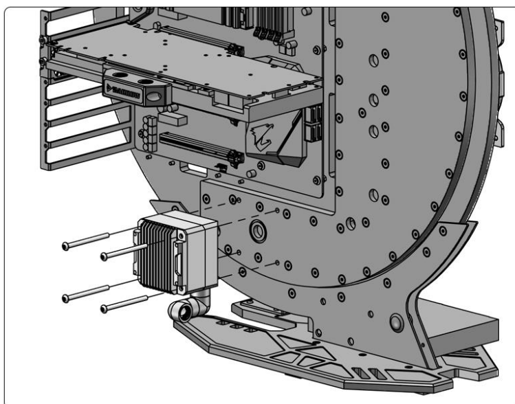
13.固定水泵
