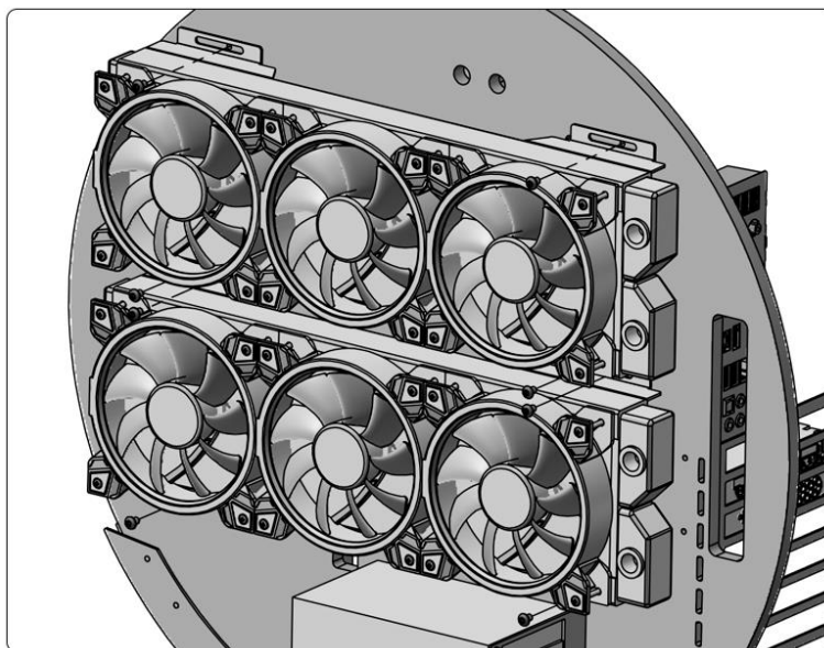
11.冷排支架固定到机箱
